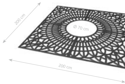
GRILLE 1A GR-KW-001
