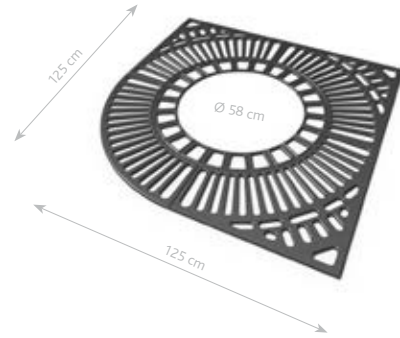
GRILLE MIX 1 GR-KW-015
