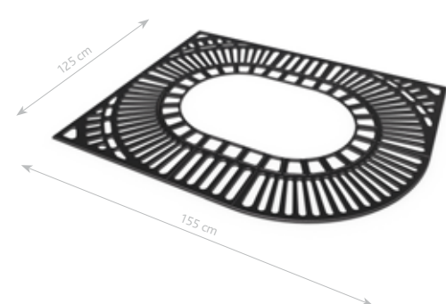
GRILLE MIX 6 GR-KW-020
